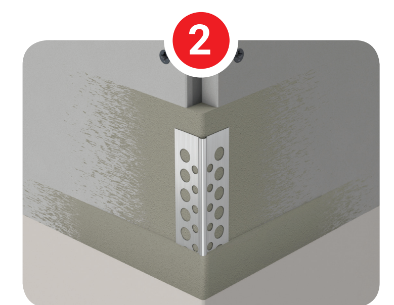
PC X04AL alumīnija stūra profils, punktots
