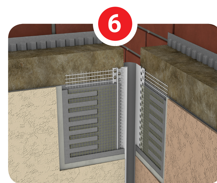
EM V40 deformācijas šuvju profils stūrim, 2.5 m
