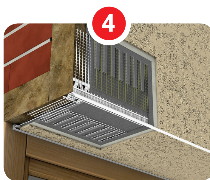
ED C 01 stūra profils ar lāseni, 2.5 m
