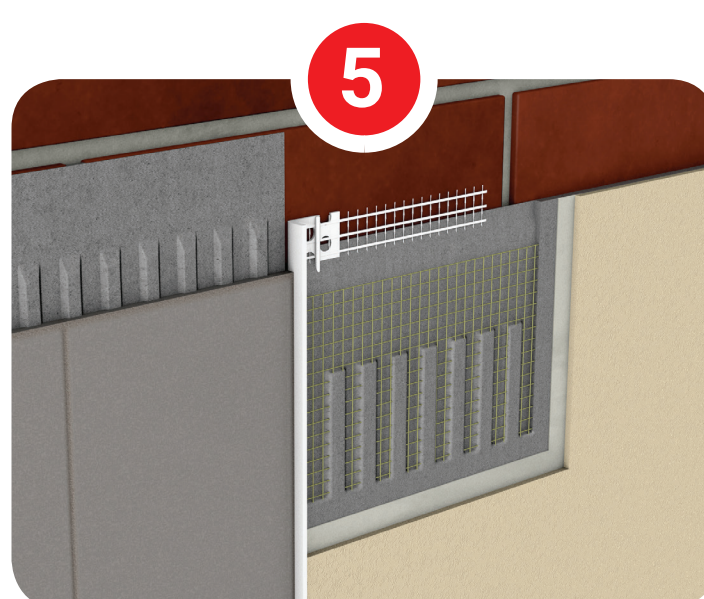
EST nobeiguma / turpinājuma profils
