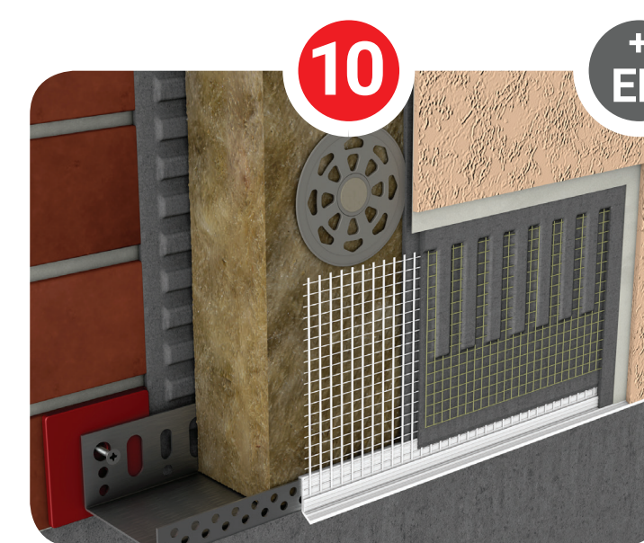
ED BK papildus lāsenis ar sietu (uzspraužams) cokola profilam
