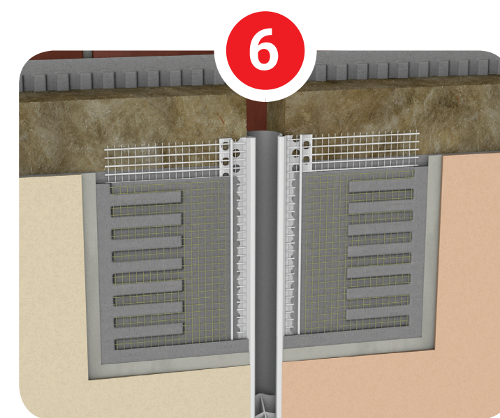
EM E40 deformācijas šuvju profils plaknei, 2.5 m
