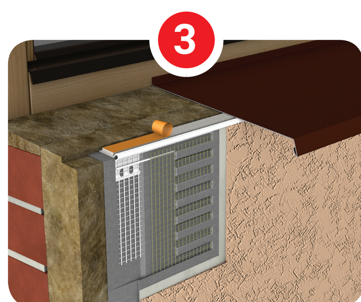
EW US 01 palodzes montāžas profils 90° – 130°, 2.0 m
